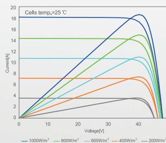
不同辐照度下电流电压曲线 / 功率电压曲线 (720W)
