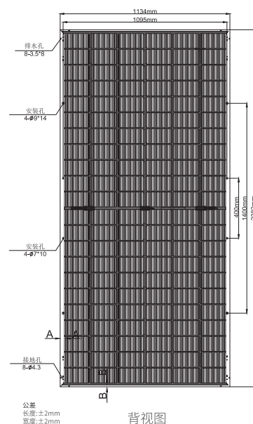
背视图
