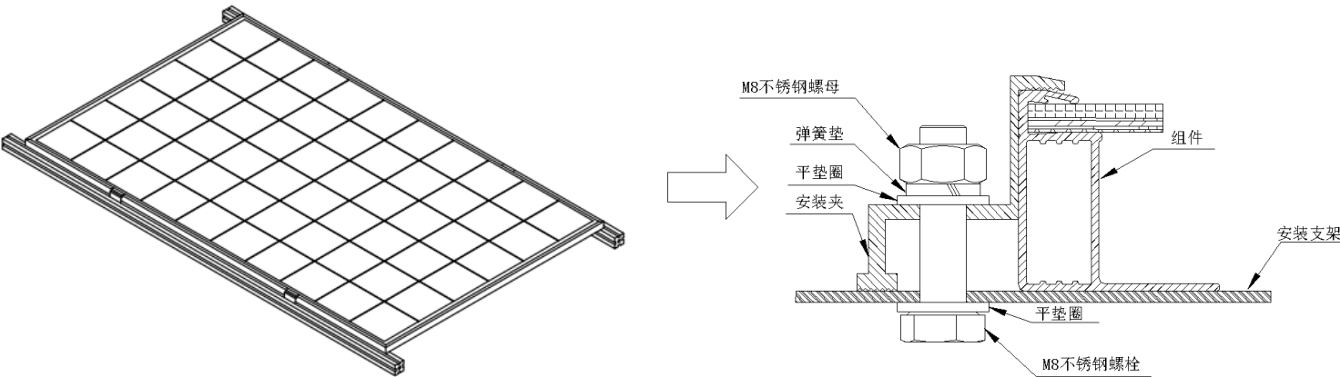
图 6 安装夹安装
