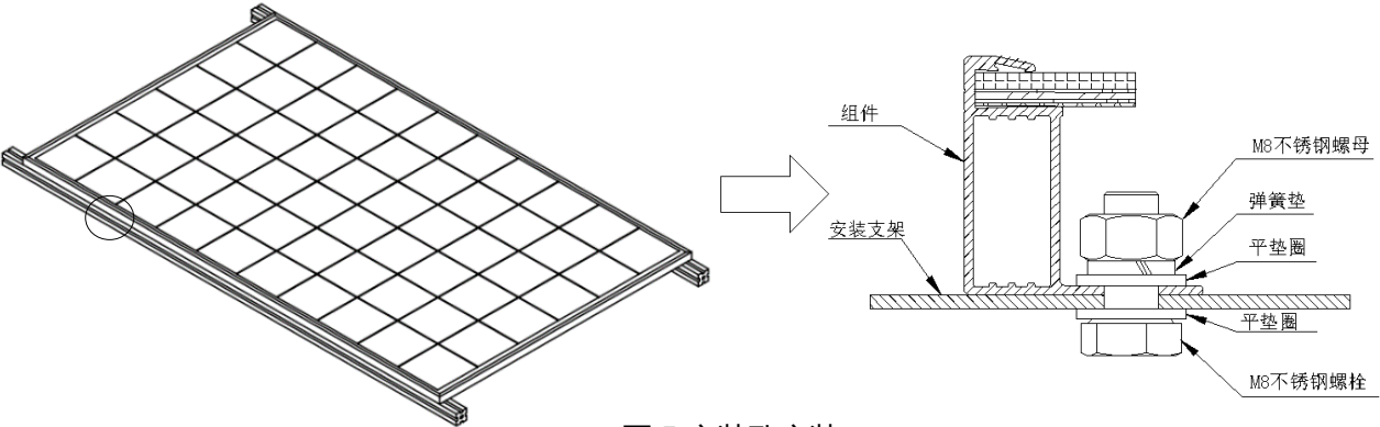
图 5 安装孔安装
